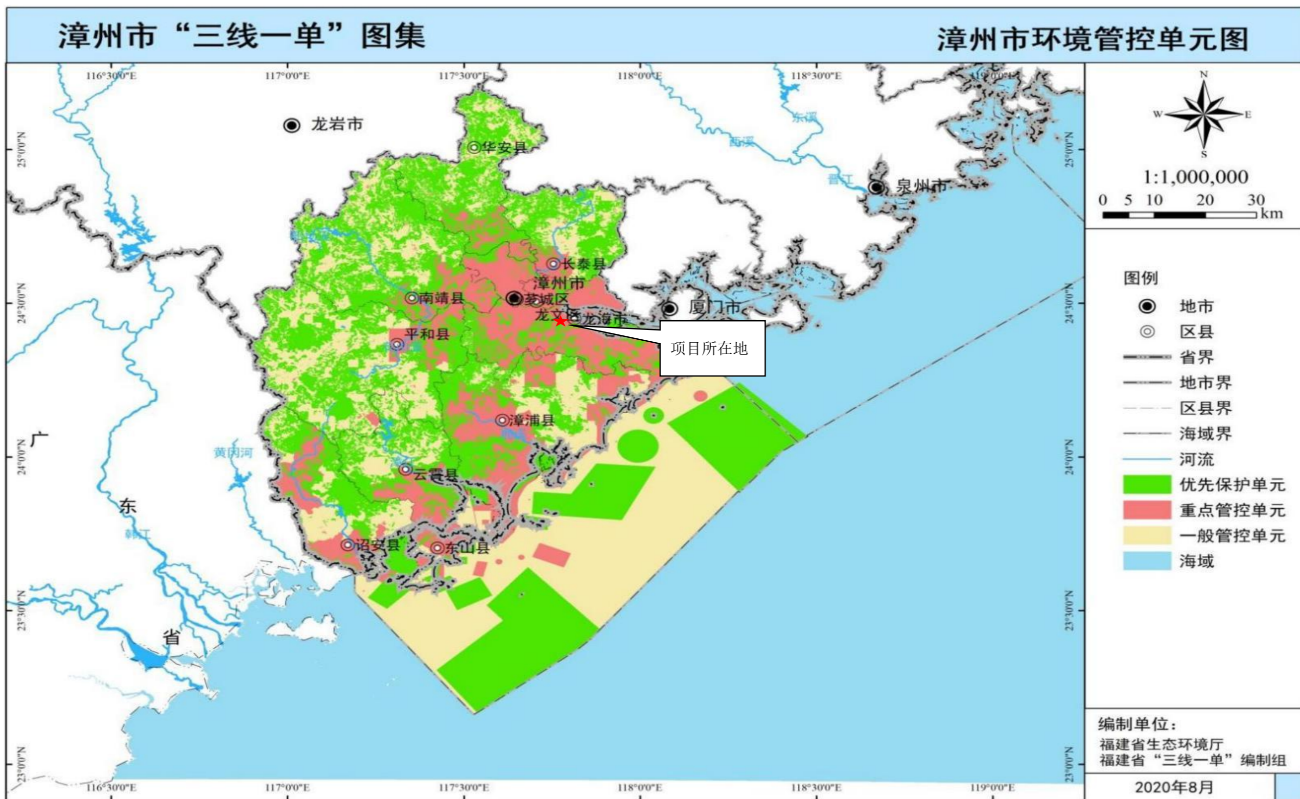
附图6 漳州市环境管控单元图
